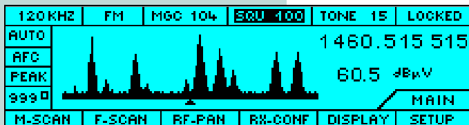
IF panorama
